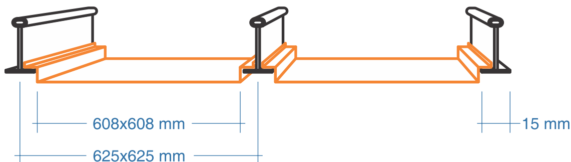
Forro Zimplac Perfurado Ø2,5mm Referencia: 2555 Área perfurada: 16%
